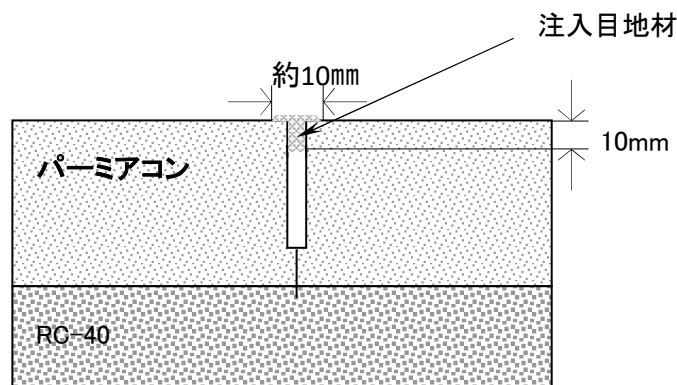
収縮目地の断面図 (カッター幅 3mm程度)
