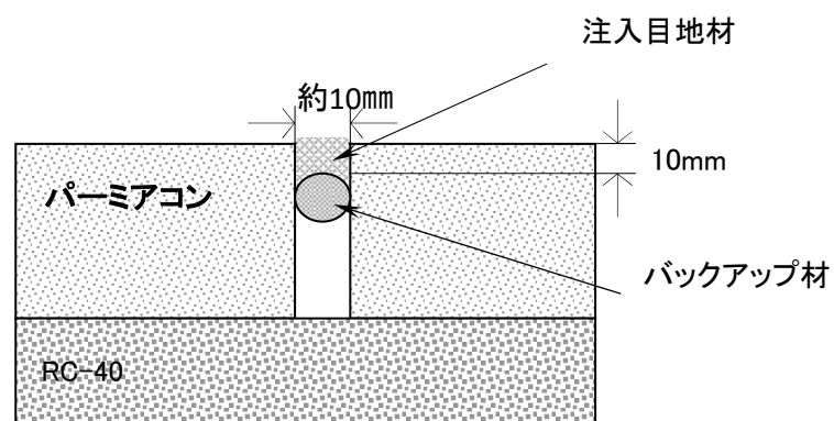
膨張目地の断面図 (カッター幅 8mm程度)
